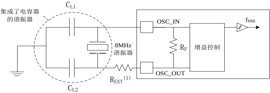
图 14 使用 8MHz 晶体的典型应用
