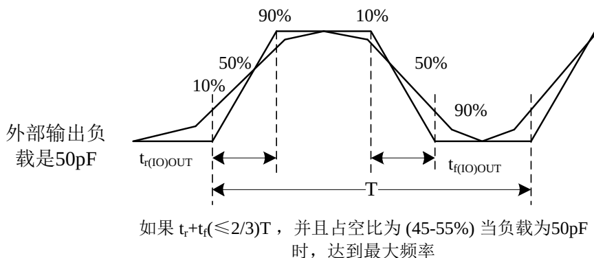
图 18 输入输出交流特性定义
