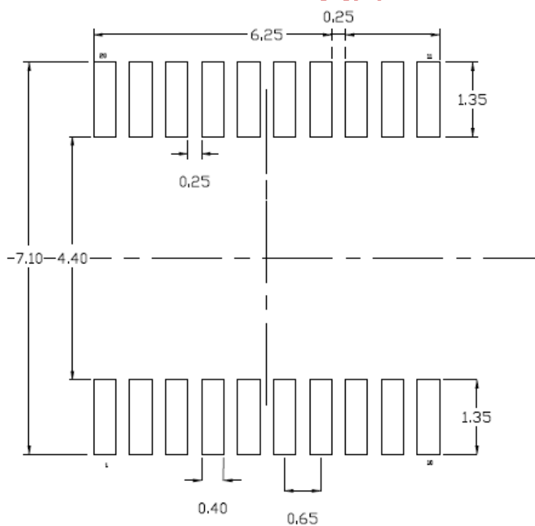
图 32 TSSOP20 推荐封装
