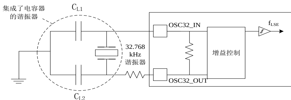
图 15 使用 32.768kHz 晶体的典型应用
