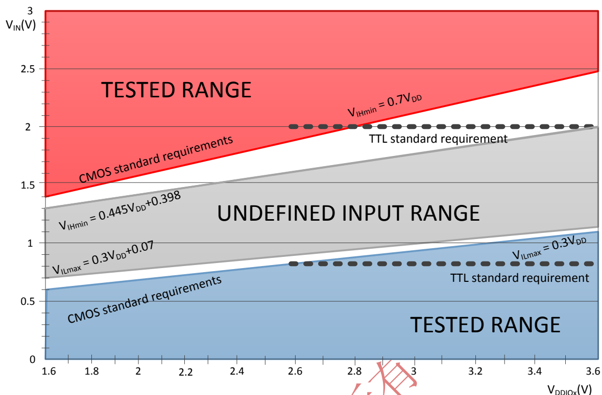
图 16 TC 和 TTa 的 I/O 口输入特性
