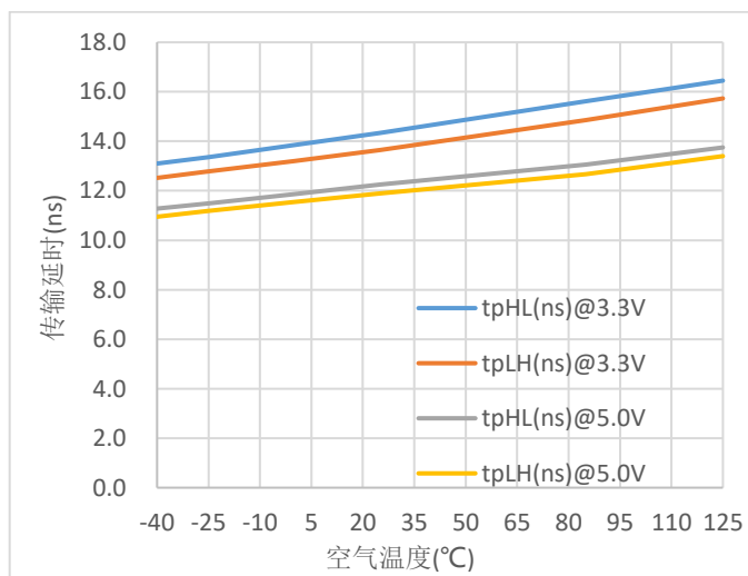
图 12. \pi 12\text{xM}6\text{x} 传输延时 vs. 空气温度
