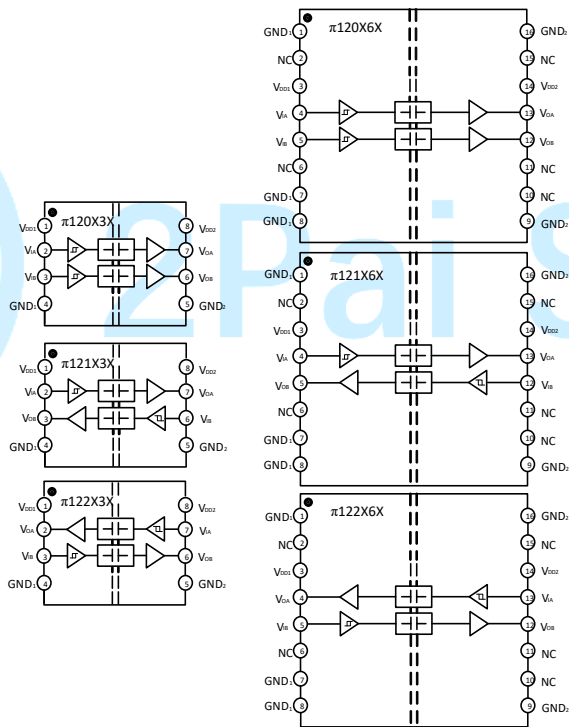
图 1. \pi 120xxx/\pi 121xxx/\pi 122xxx 功能框图
