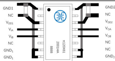
图 15.推荐的印刷电路板布局
