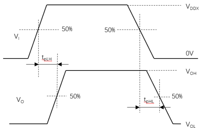
图 14. 传输延迟时间波形测量
