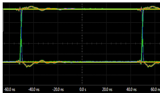
图 16. \pi 12 \times M \times X 眼图
