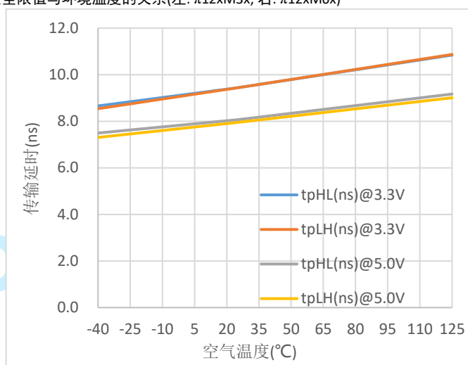
图 11. \pi 12\text{xM}3\text{x} 传输延时 vs. 空气温度
