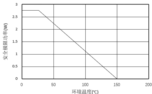
图 9.热降额曲线, 依据 DIN V VDE V 0884-10 的安全限值与环境温度的关系(左: \pi 12\text{xM}3\text{x} ; 右: \pi 12\text{xM}6\text{x} )
